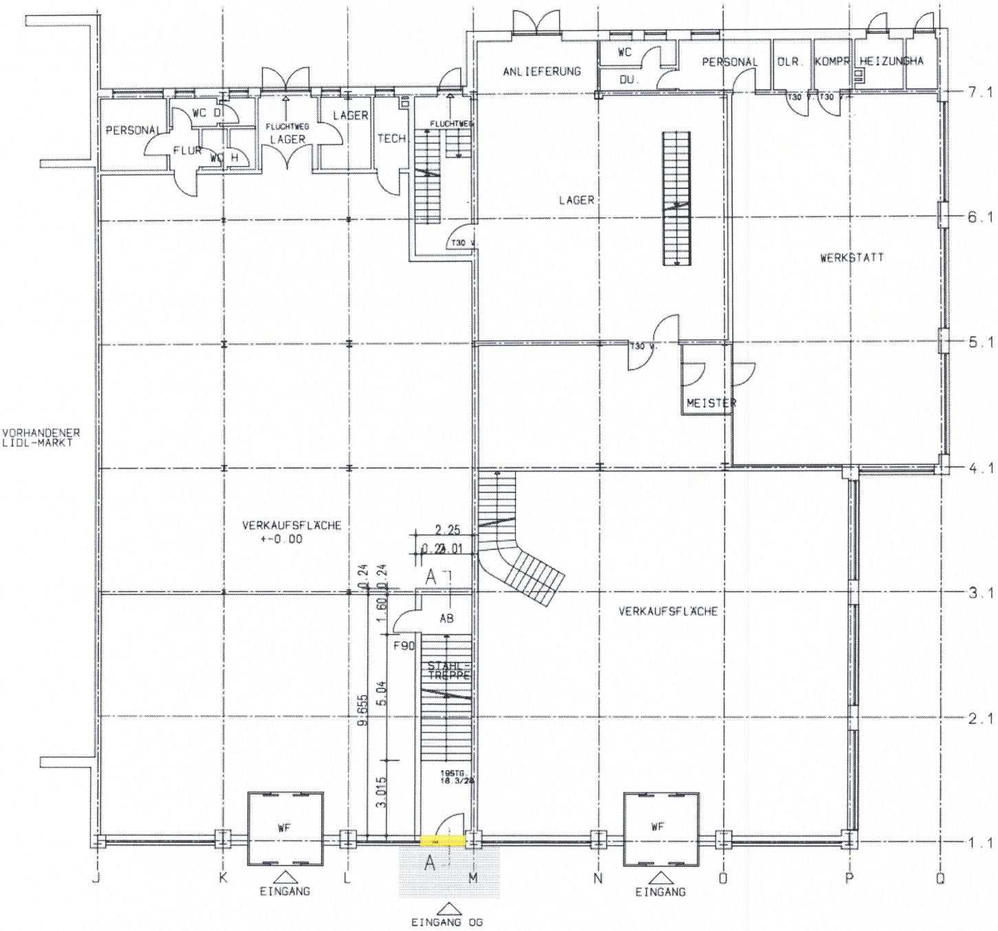
ERDGESCHOSS
