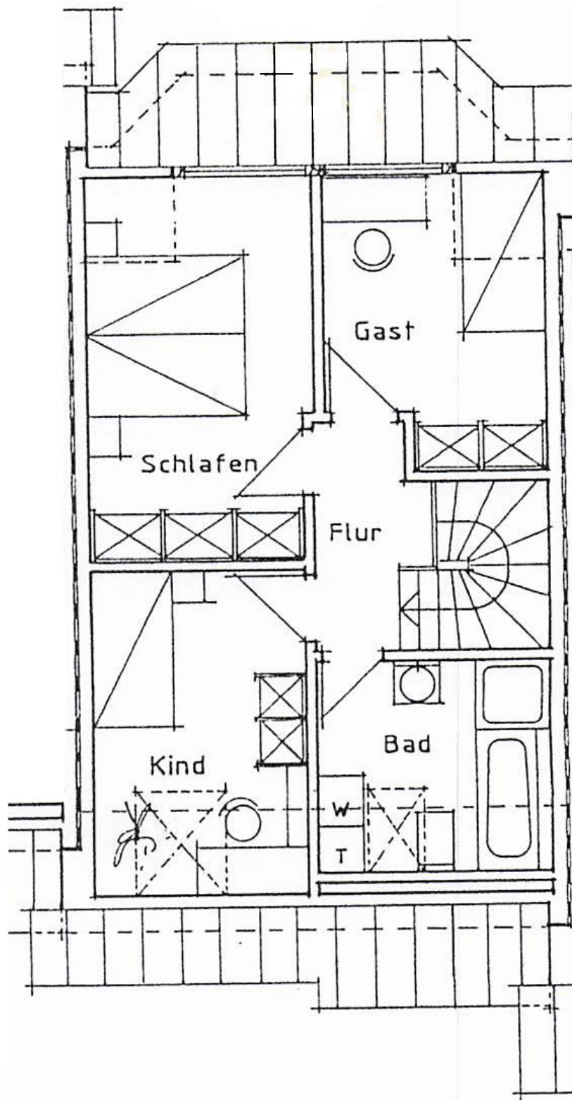
Grundriss Obergeschoss
